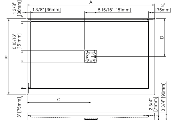
EN COIN MUR À GAUCHE (L)
