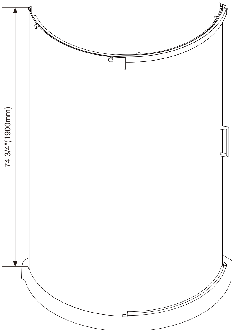
DESSIN PORTE DROITE/DRAWING RIGHT DOOR
